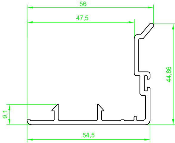
(ST 7210)"SÜRMETEC" Yeni Kilitleme Profili Ö:1/1 (ST 7210) "SURMETEC" New İnterlocking Profile S:1/1
