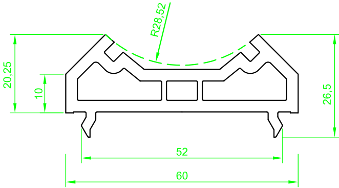
(ST 6900)"STARTEC" Köşe Dönüş Adaptörü Ö:1/1 (ST 6900) "STARTEC" Corner Adapter S:1/1
