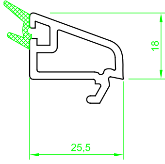
(ST 7450)"SÜRMETEC" Yapıştırma Contalı Tek Cam Çıtası Ö:1/1 (ST 7450) "SURMETEC" Co Extruded Rustick Single Glazing Bead S:1/1
