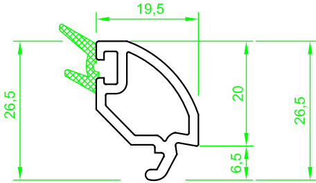
(ST 6650) "MEGATEC" Contalı Çift Cam Çıtası " (ST 6650) "MEGATEC" Double Glazing Bead"
