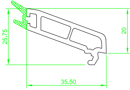
(ST 6520) "STARTEC" Yap.Contalı Tek Cam Çıtası Ö:1/1 (ST 6520) "STARTEC" Co-Extruded Single Glazing Bead S:1/1
