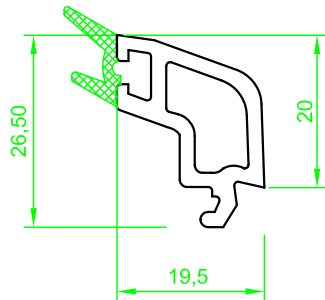
(ST 6640) "STARTEC" Çift Cam Çıtası Ö:1/1 (ST 6640) "STARTEC" Double Glazing Bead S:1/1
