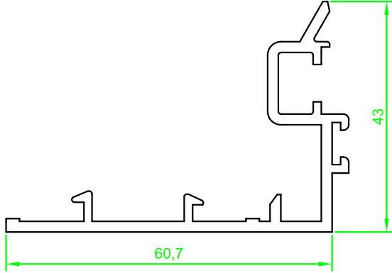
(ST 7200)"SÜRMETEC" Kilitleme Profili Ö:1/1 (ST 7200) "SURMETEC" İnterlocking Profile S:1/1
