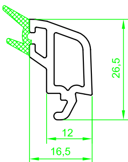
(ST 6630) "STARTEC" 24mm Yap. Contalı Çift Cam Çıtası Ö:1/1 (ST 6630) "STARTEC" Co-Extruded Double Glazing Bead 24mm S:1/1
