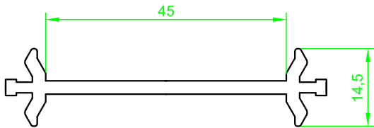
(ST 6920)"STARTEC" I Bağ Profili Profili Ö:1/1 (ST 6920) "STARTEC" I Coupling Profile S:1/1
