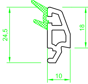
(ST 7460)"SÜRMETEC" Yapıştırma Contalı Çift Cam Çıtası Ö:1/1 (ST 7460) "SURMETEC" Co Extruded Rustick Double Glazing Bead S:1/1
